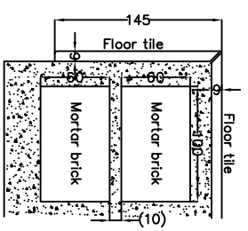
B-B Section enlargement
